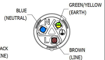
VDE WIRING
